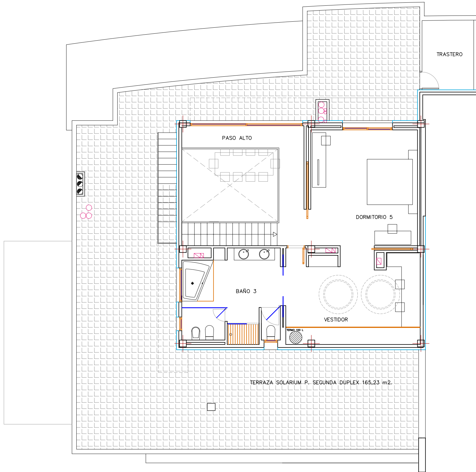
PLANTA SEGUNDA DUPLEX
