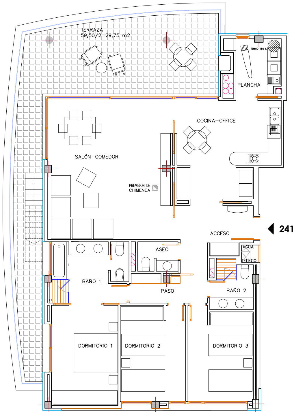
PLANTA CUARTA
